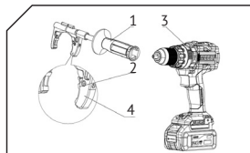
1 - Рукоятка; 2 - Штифт; 3 - Место установки с пазами; 4 - Крепление
