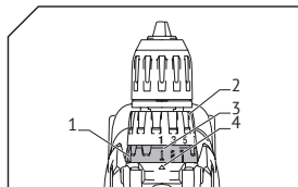
1 - Кольцо выбора режима работы; 2 - Кольцо регулировки крутящего момента; 3 - Режим; 4 - Указатель
